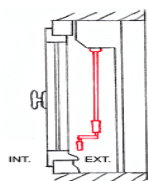
Tringle oscillante sortie sous caisson
